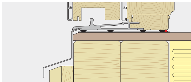
Skjurdörr tröskel Trägol
