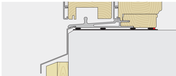
Skjurdörr tröskel platta på mark
